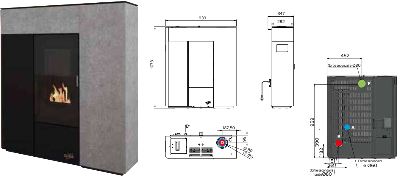
Version sortie dessus concentrique (Réf. ORVAL SDC)
